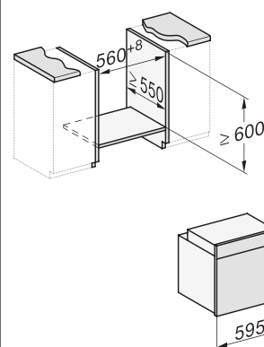
Einbau im Unterschrank
